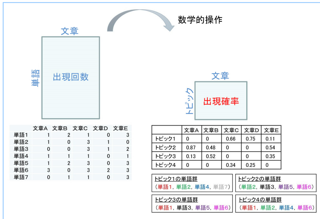
図2 潜在的な意味情報の抽出
