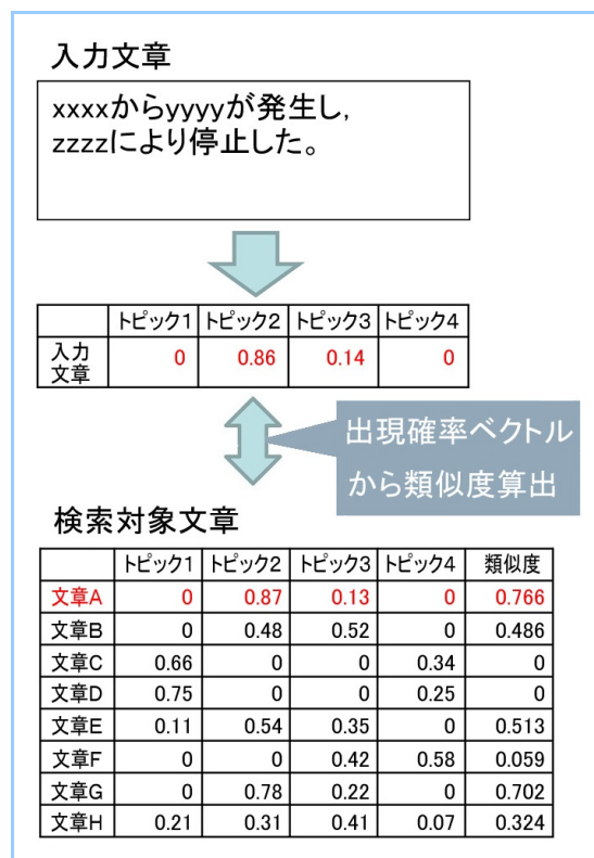
図4 入力文章に対する類似度算出
