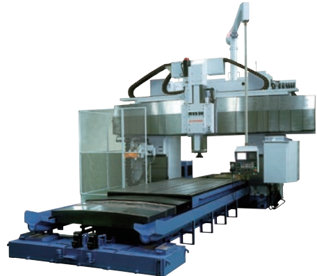
門形五面加工機 MVR30
