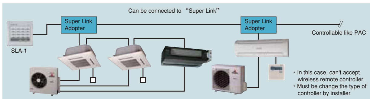
図 1 スーパーリンクとの接続概念図
