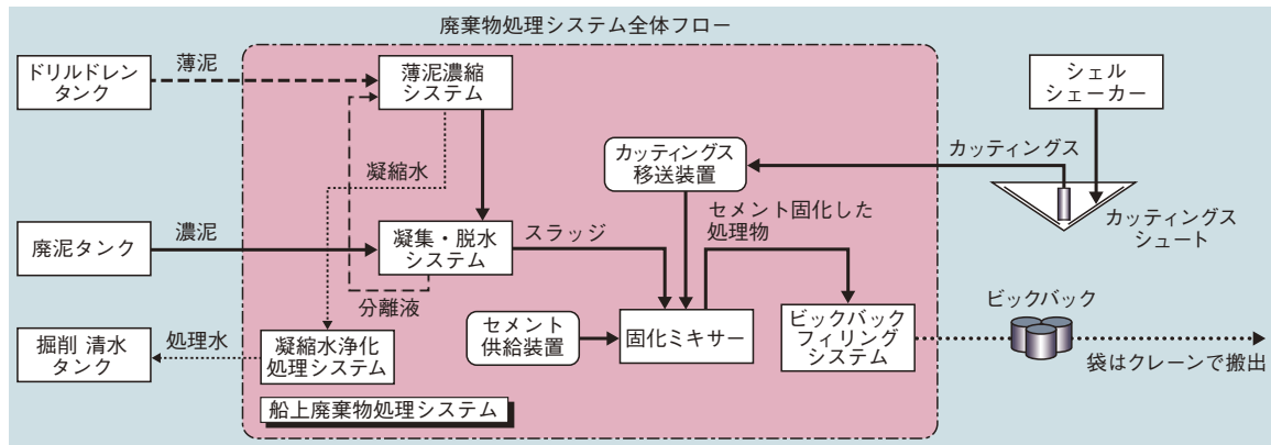
図3 廃泥水処理システム全体フロー
