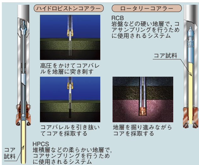
図2 HPCS と RCB
