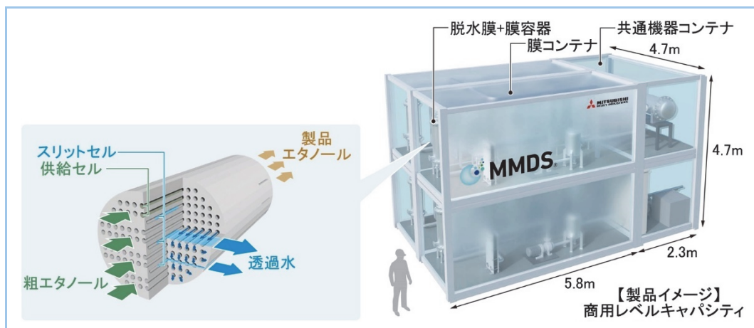
図4 商用機イメージ
