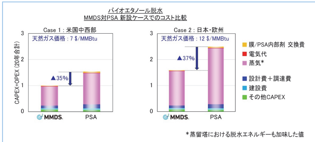
図3 膜分離脱水システムと PSA の経済性比較
