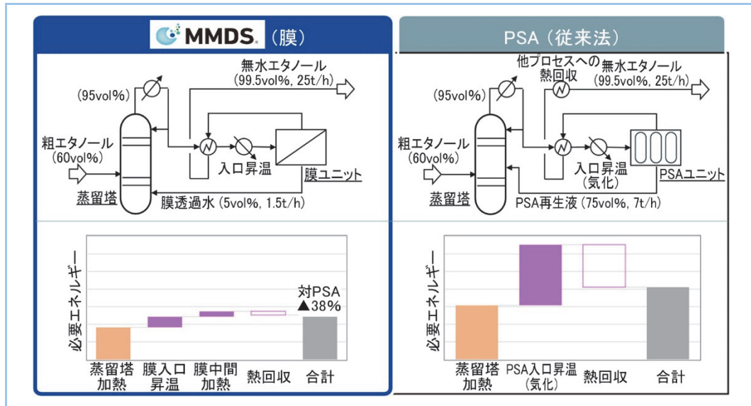
図2 必要脱水エネルギーの比較
