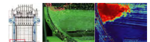
原子炉模型内の流動評価（速度、温度の同時計測）
