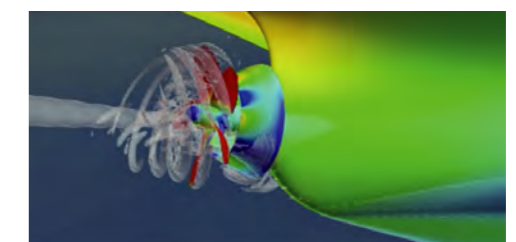
プロペラ周りの流場計算（圧力分布と渦の可視化）
