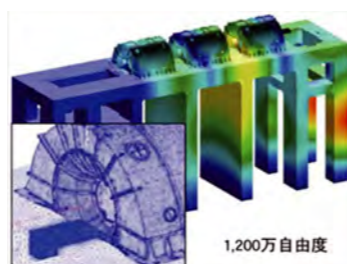
架台・車室・軸の連成振動解析 1,200万自由度
