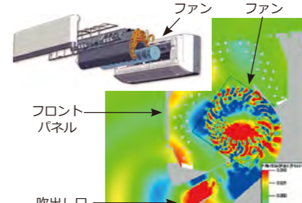
流体力学解析技術
