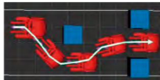
移動体の障害物回避最適経路計画
