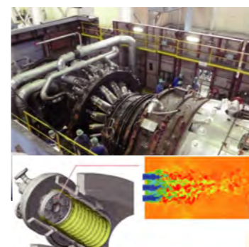
水素GT燃焼器と燃焼解析
