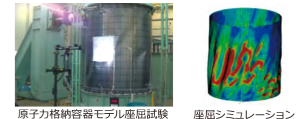
原子力格納容器モデル屈曲試験
