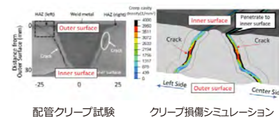
配管クリープ試験
