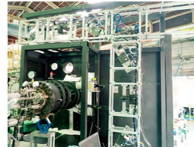
ガスタービン 大気圧燃焼試験 火炎3次元CT装置
