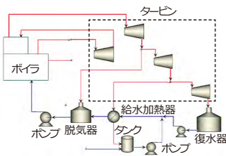
熱サイクル解析技術
