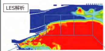
LES解析
