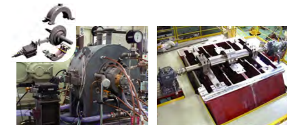
高速回転シール試験機 (max15,000rpm)
