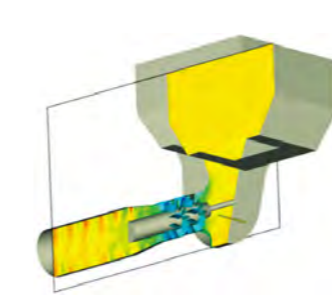
低騒音軸流ファンの開発
