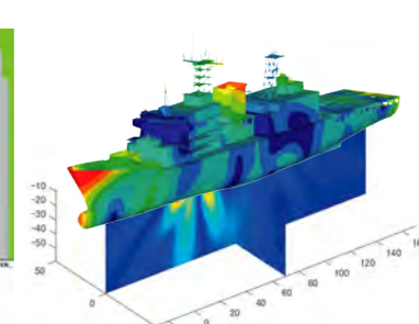
船舶騒音・振動解析
