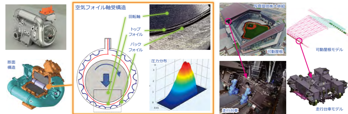
燃料電池車用電動コンプレッサ向け 空気フォイル軸受の特性解析
