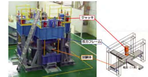
原子炉における加圧熱衝撃模擬試験装置
