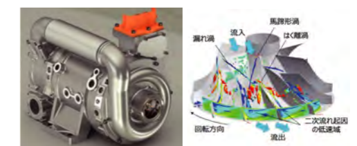
エアコンプレッサ
