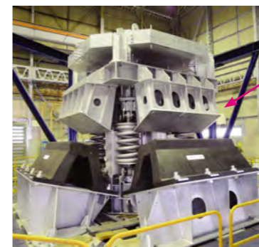
東京スカイツリー風揺れ用制振装置の性能検証
