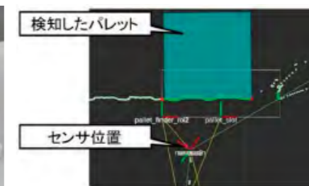
LiDARによるパレットの検出・位置推定
