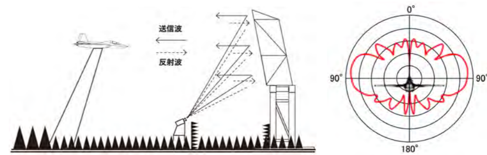
電波特性評価試験
