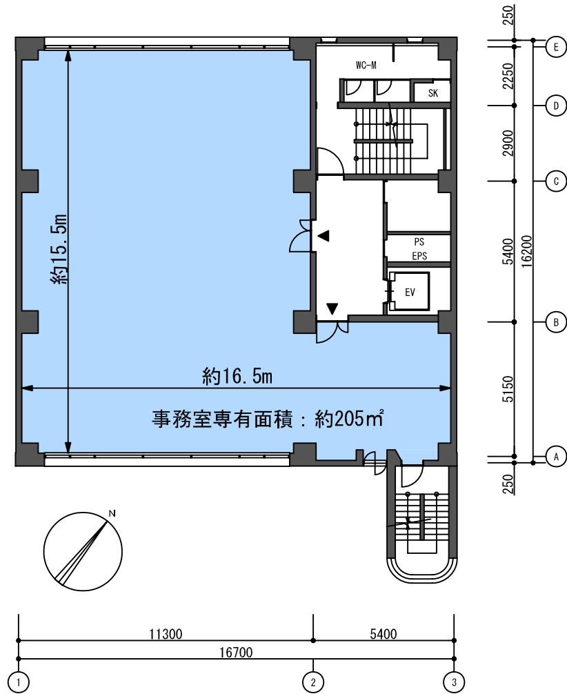
第四田町ビル 基準階平面図
