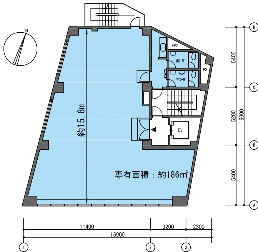
芝サエスワカマツビル 基準階平面図
