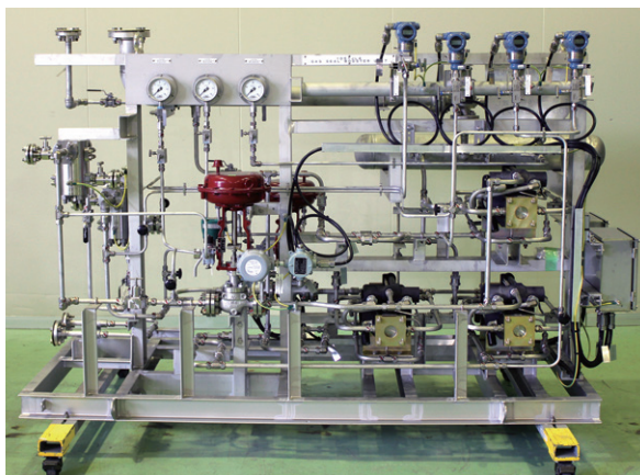
高圧ガス昇圧装置
