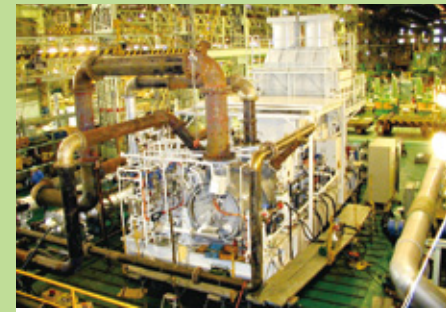
F 洋上ガス処理設備用圧縮機
