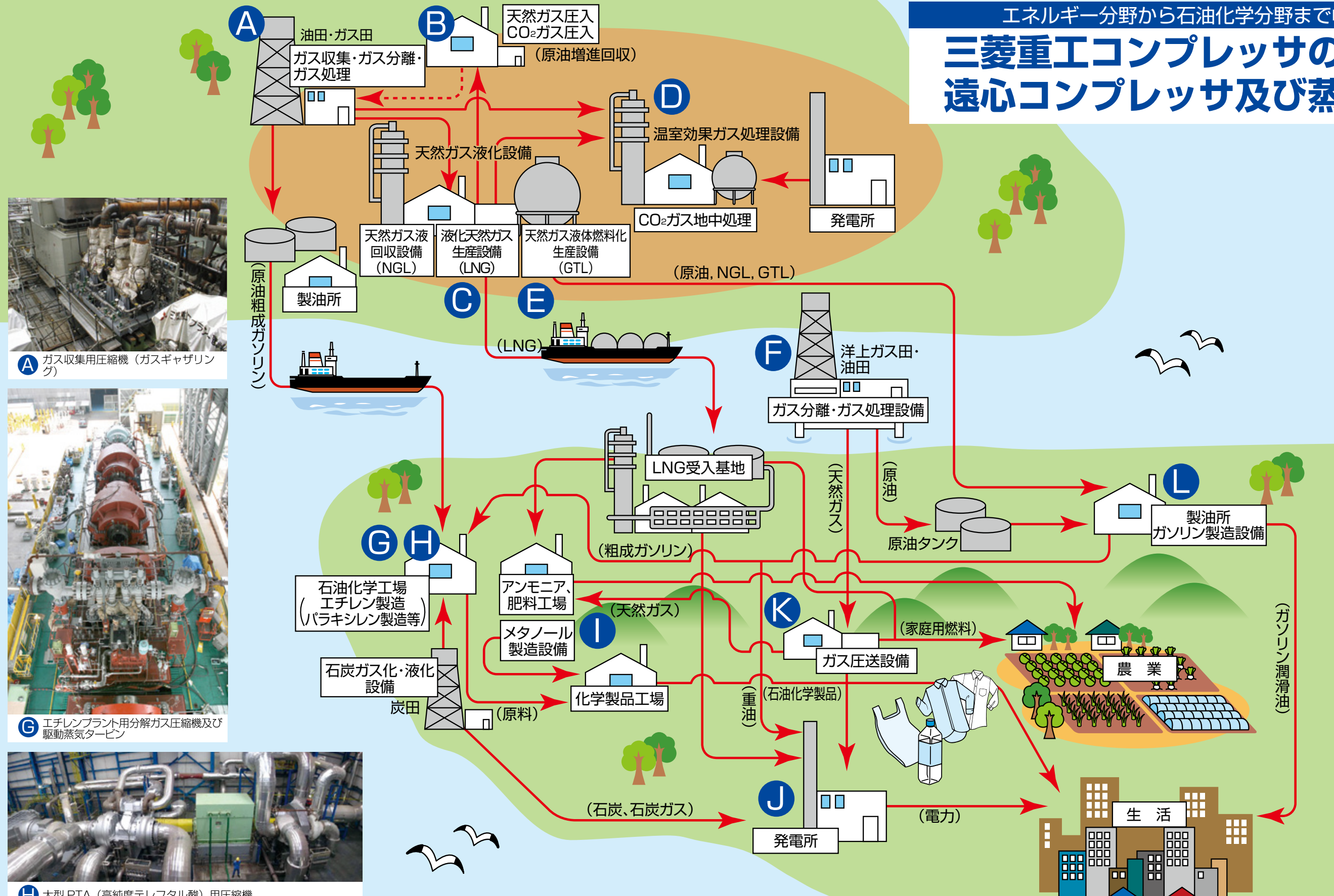
H 大型 PTA (高純度テレフタル酸) 用圧縮機
