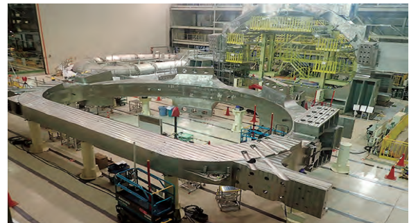
国際熱核融合実験炉 超電導コイル
