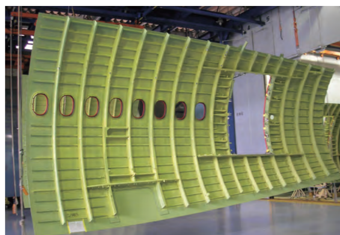
胴体パネル完成品（内側）
